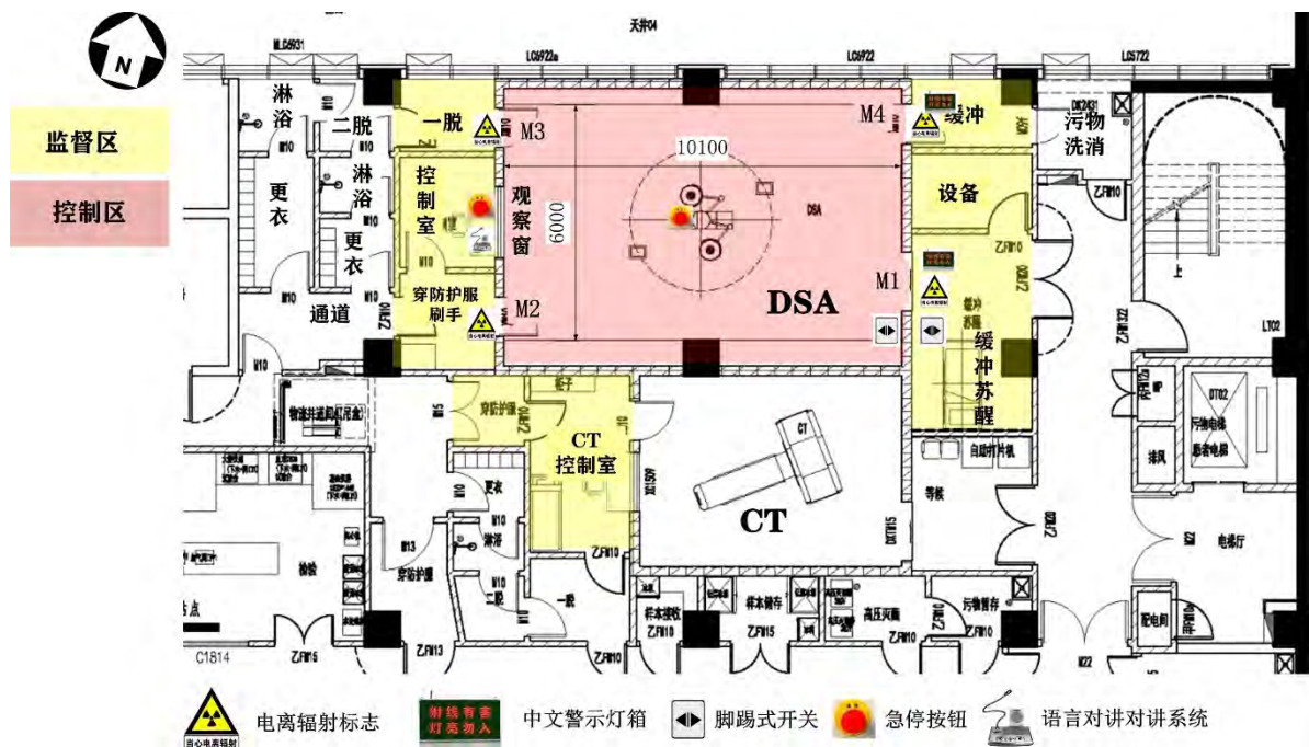
图 10-1 DSA 手术室辐射安全与防护设施布置示意图
