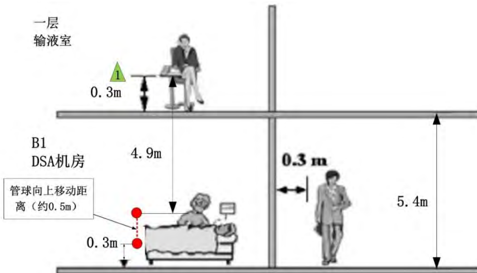
图 11-4 DSA 手术室估算点位置剖面示意图
