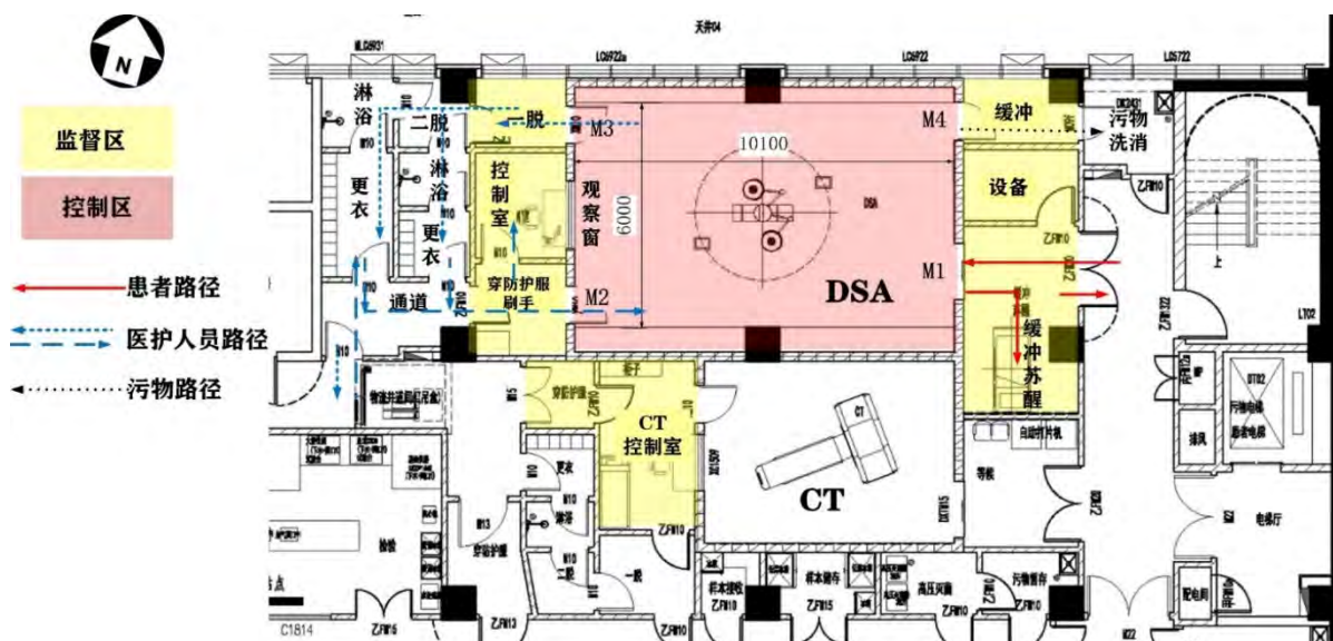
图 11-1 发热门诊楼地下一层 DSA 手术室布局、分区和路由示意图
