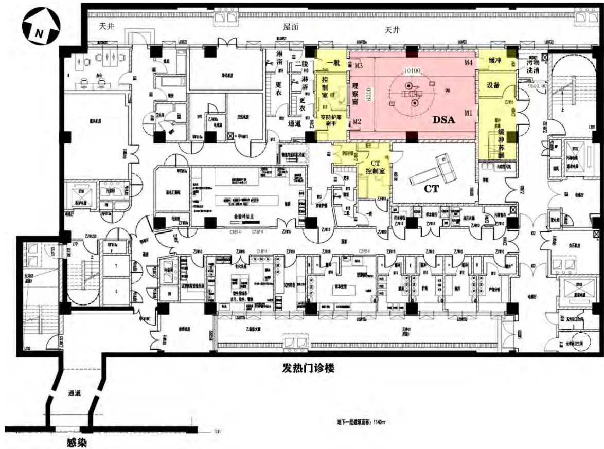
图 7-2 发热门诊楼地下一层布局和拟建 DSA 手术室位置示意图
