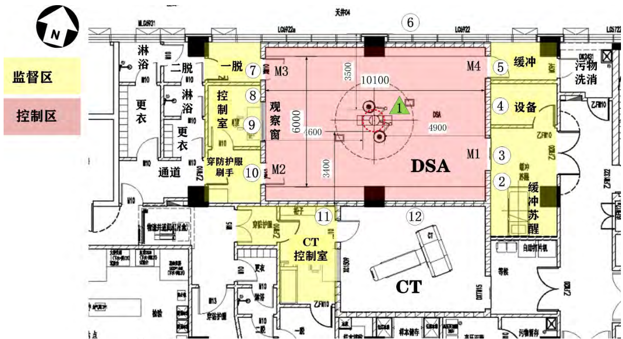
图 11-3 DSA 手术室估算点位置平面示意图
